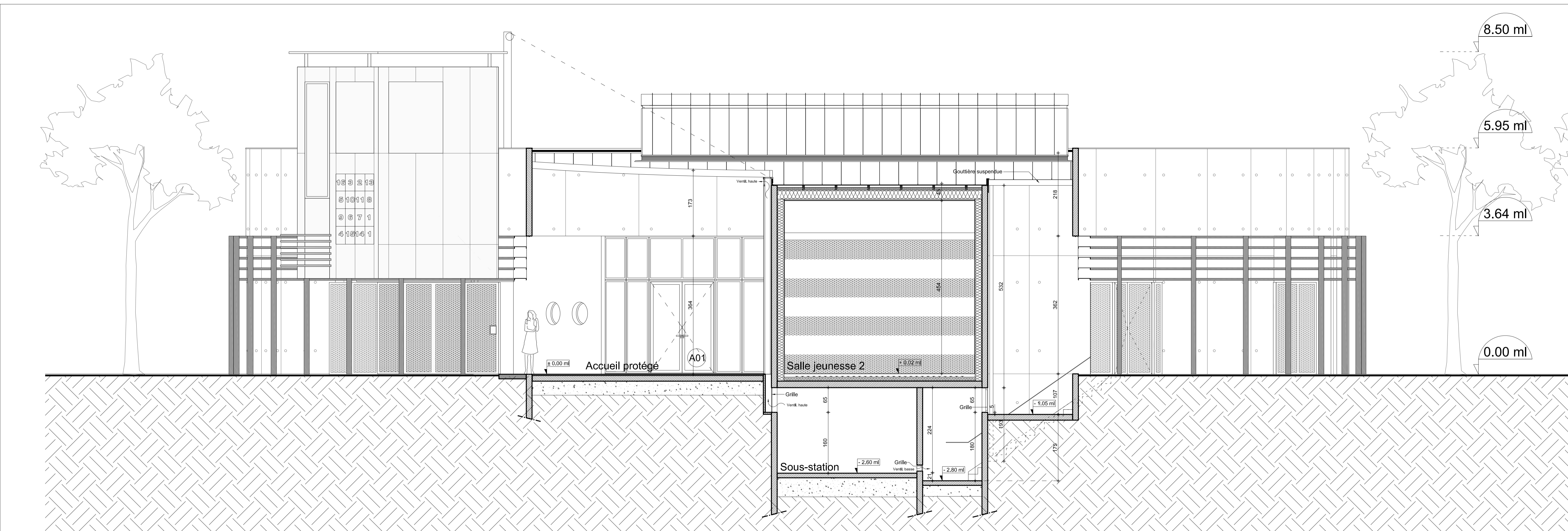
COUPE CC : Coupe sur la sous-station
