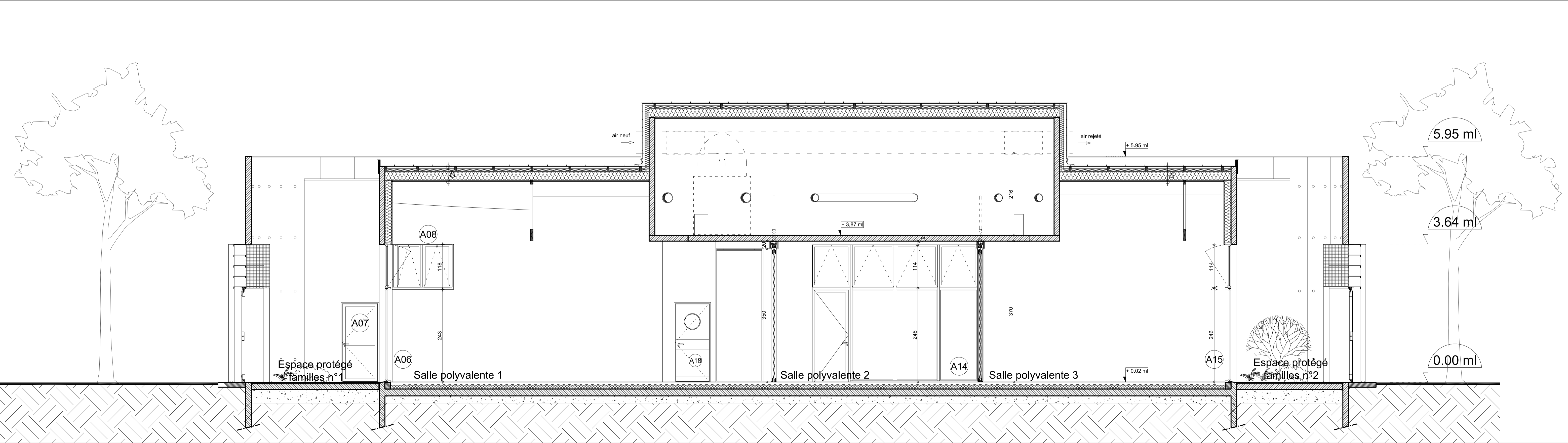
COUPE DD : Coupe sur les salles d'activités
