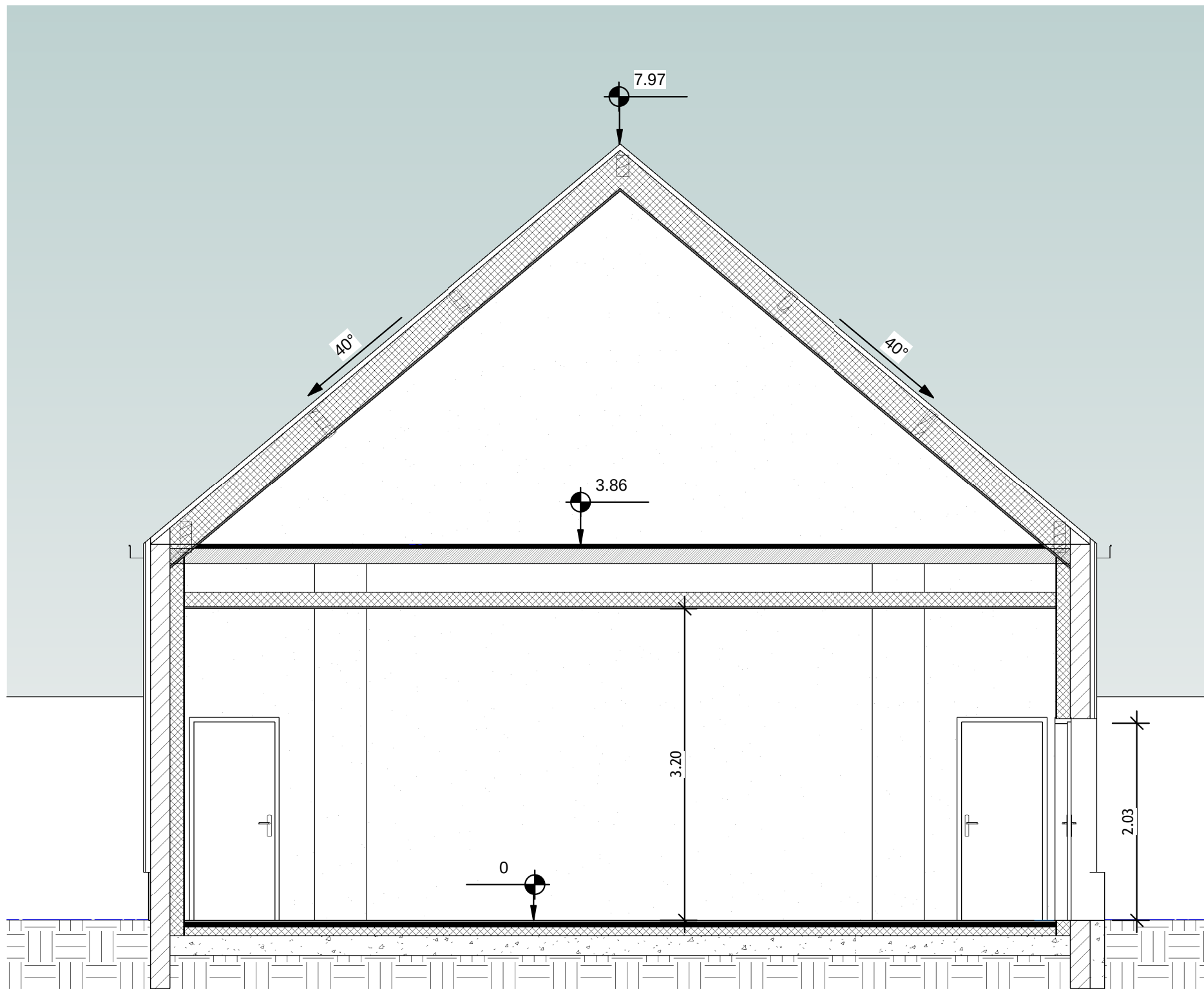
② COUPE SUR LOCAL CTA
