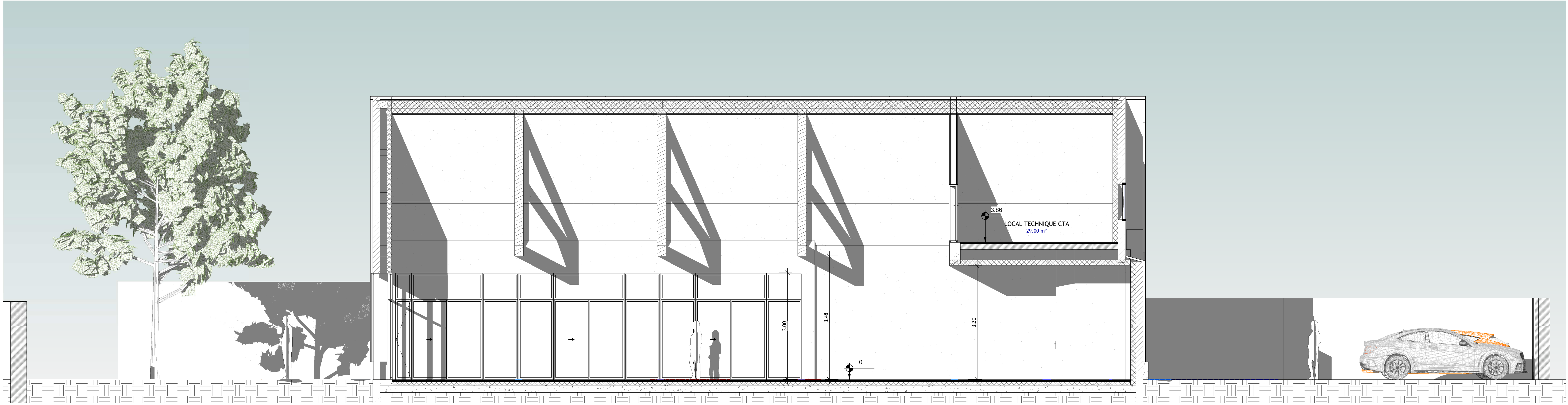
① COUPE LONGITUDINALE SALLE ASSOCIATIVE
