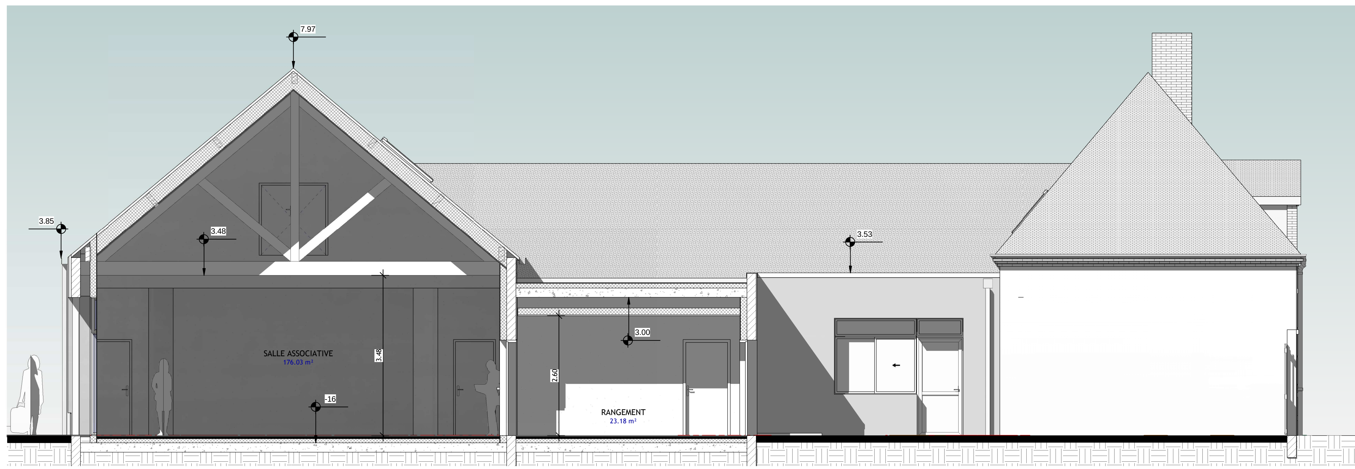
③ COUPE SUR COUR DE SERVICE
