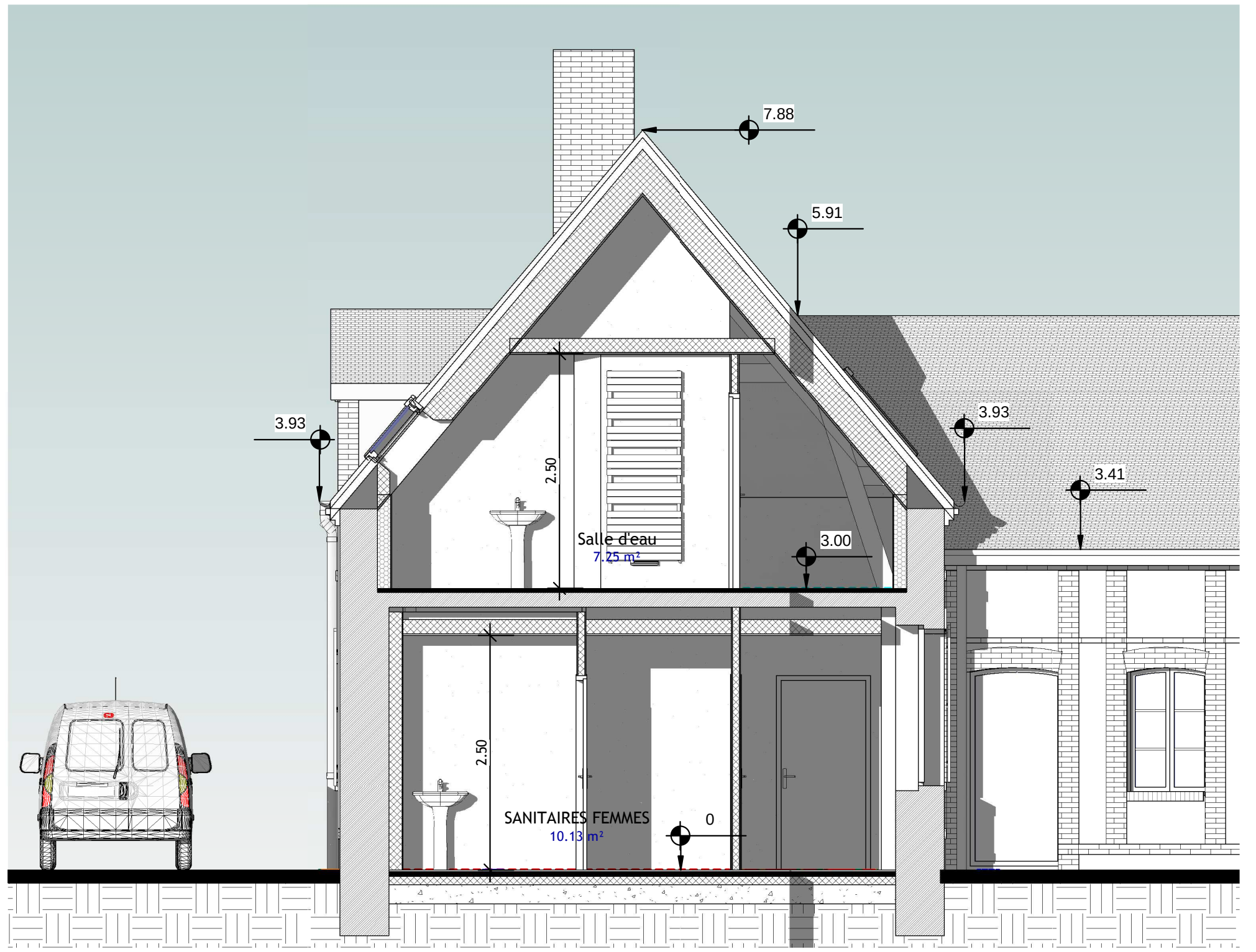
⑤ COUPE SUR BATIMENT ANCIEN
